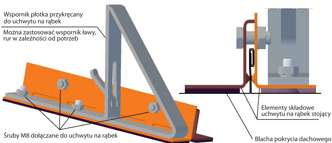
Schemat poglądowy montażu wsporników płotka i ławy na uchwycie na rąbek stojący.
